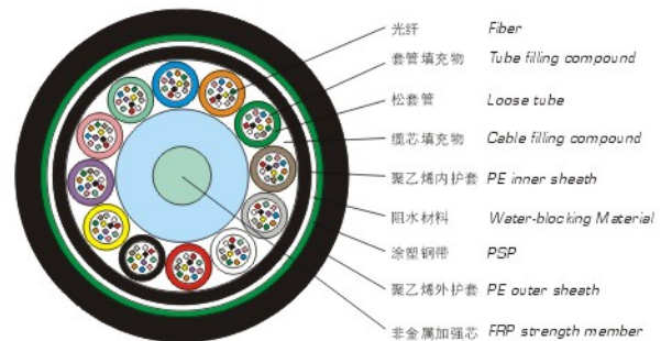
光缆结构图 Cable Structure
